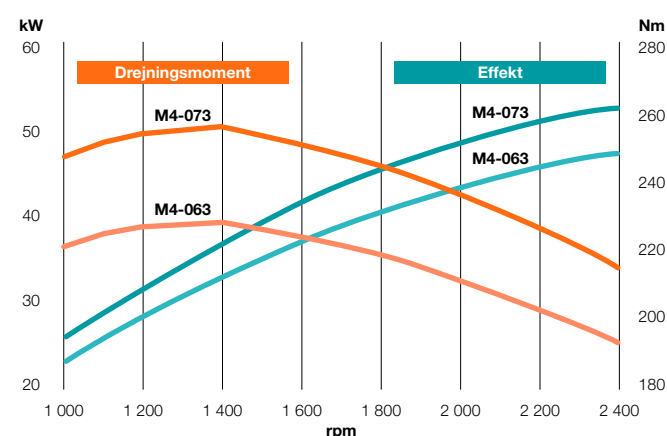
Effekt og drejningsmoment kW
